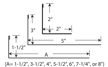
22. Angle Trim
